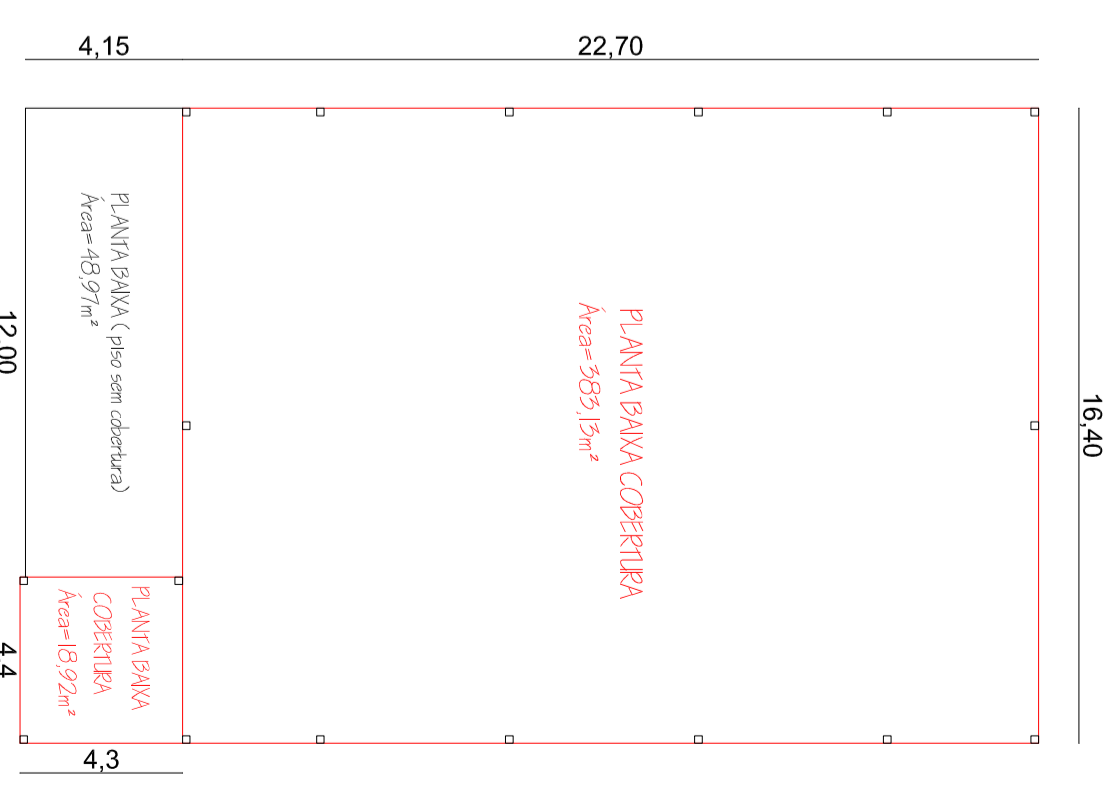
PLANTA BAIXA A total = 452,68m 2
